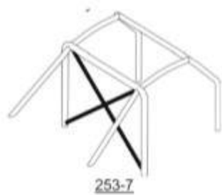
Dibujo del tirante diagonal
