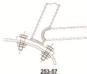
Dibujo que muestra como atornillar la placa de fijación
